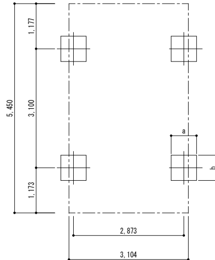
■基礎配置図
